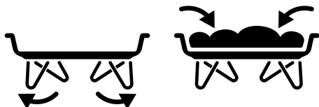
Animacja pokazująca, kiedy należy rozłożyć nóżki brytfanny
