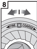
8 Verstellbaren oberen Kegel, um 1 Nummer, gröber oder feiner verschieben
